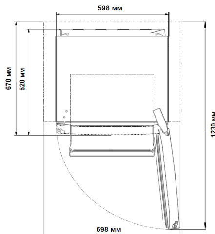
Рабочие габариты холодильного прибора.
